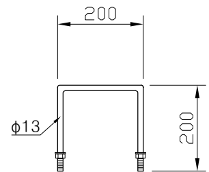
取手金具 溶接亜鉛めっきHDZ 35
