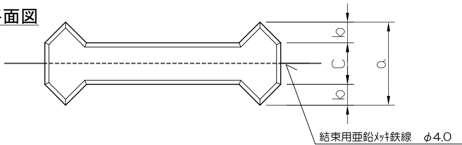
端面図
